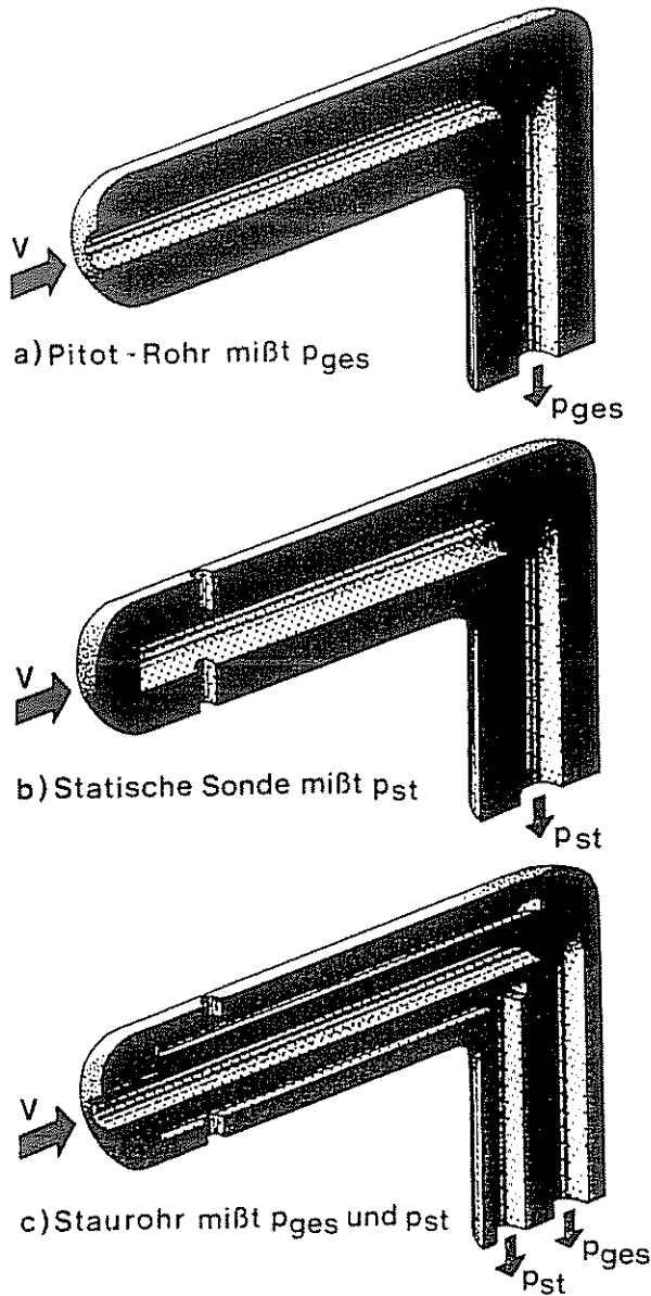
Bild 4: Sonden zu Messung von Drucken
